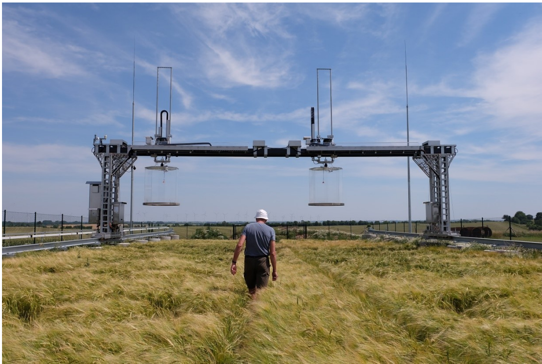
Der vom ZALF entwickelte Portalkran mit Gasmesshauben auf der CarboZALF Fläche im Landschaftslabor AgroScapeLab Quillow in der Uckermark. Mit den Hauben wird die Freisetzung von Treibhausgasen wie Kohlendioxid und Lachgas in Abhängigkeit von der Landnutzungsart bestimmt. | Foto: Julia Lidauer © ZALF | Bildquelle in Farbe und Druckqualität: http://www.zalf.de/de/aktuelles
